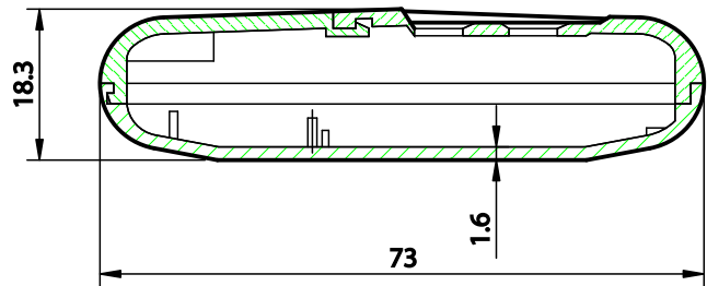
sez.A-A
